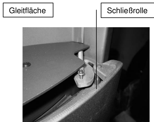
Abb. 5 (ohne Wärmefacheinlegeplatte)
